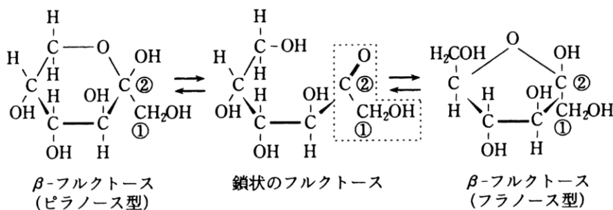
水溶液中におけるフルクトースの平衡
