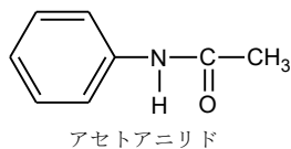
アセトアニリド
