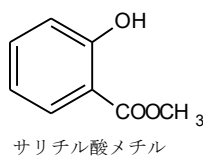
サリチル酸メチル
