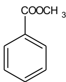
安息香酸メチル
