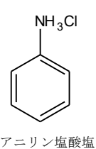
アニリン塩酸塩
