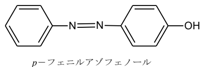
p-フェニルアゾフェノール
