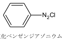
塩化ベンゼンジアゾニウム
